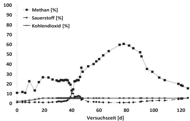
Abbildung 3: Gaskonzentrationen in Reaktor 2.
